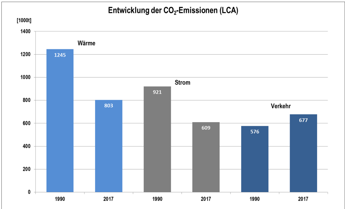
Abbildung 3: Entwicklung der CO 2 -Emissionen
