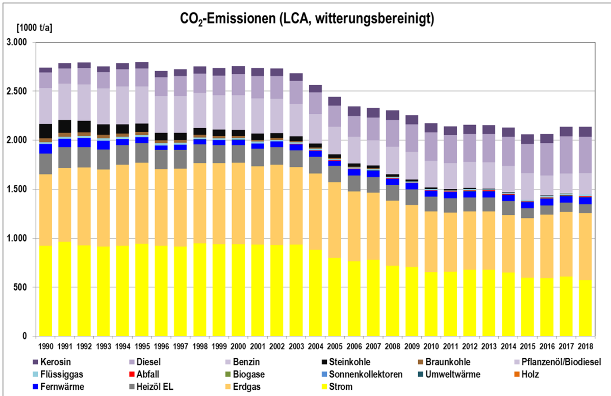
Abbildung 2: CO 2 -Emissionen auf Primärenergiebasis mit Witterungskorrektur
