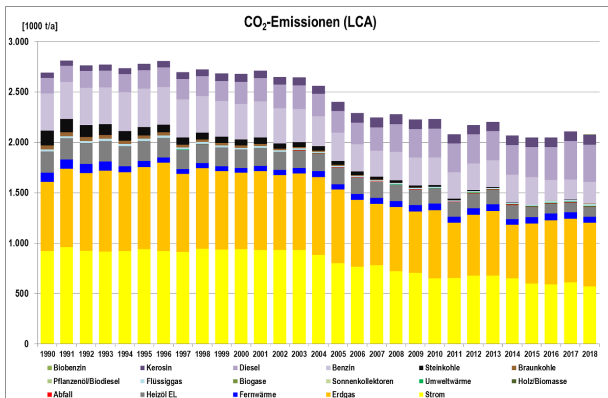
Abbildung 1: CO 2 -Emissionen auf Primärenergiebasis
