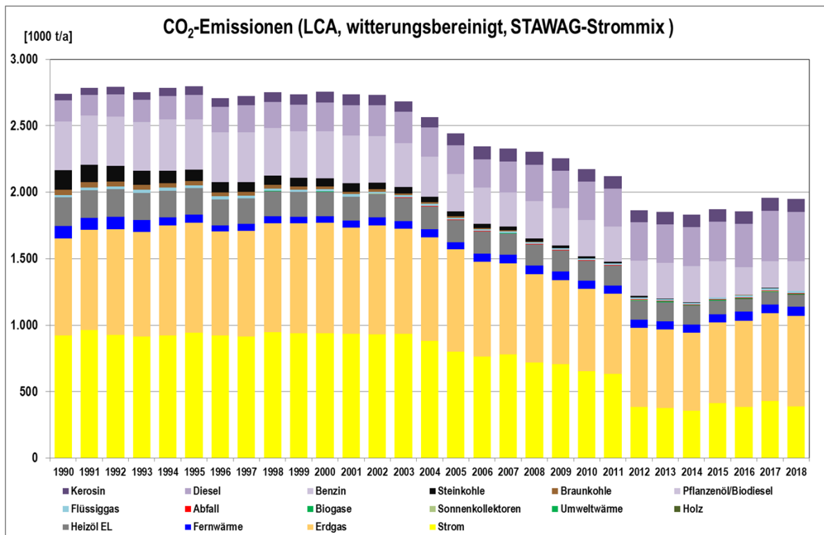
Abbildung 5: CO 2 -Bilanz bei Berücksichtigung STAWAG-Strom-Mix (seit 2012)
