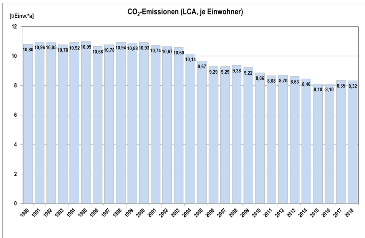
Abbildung 4: CO 2 -Emissionen / Einwohner
